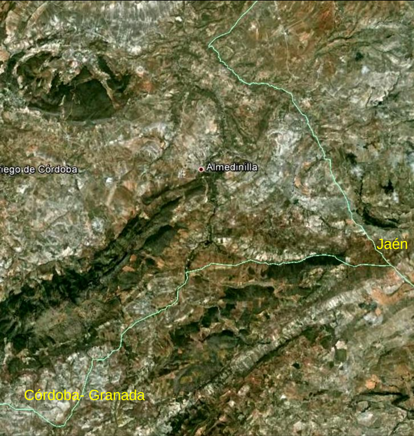
Entorno NW Hoja de Alcalá La Real, 990. Córdoba- Granada – Jaén /Arroyo al S de Almedinilla, Córdoba. (por fdo fuentes-google)
