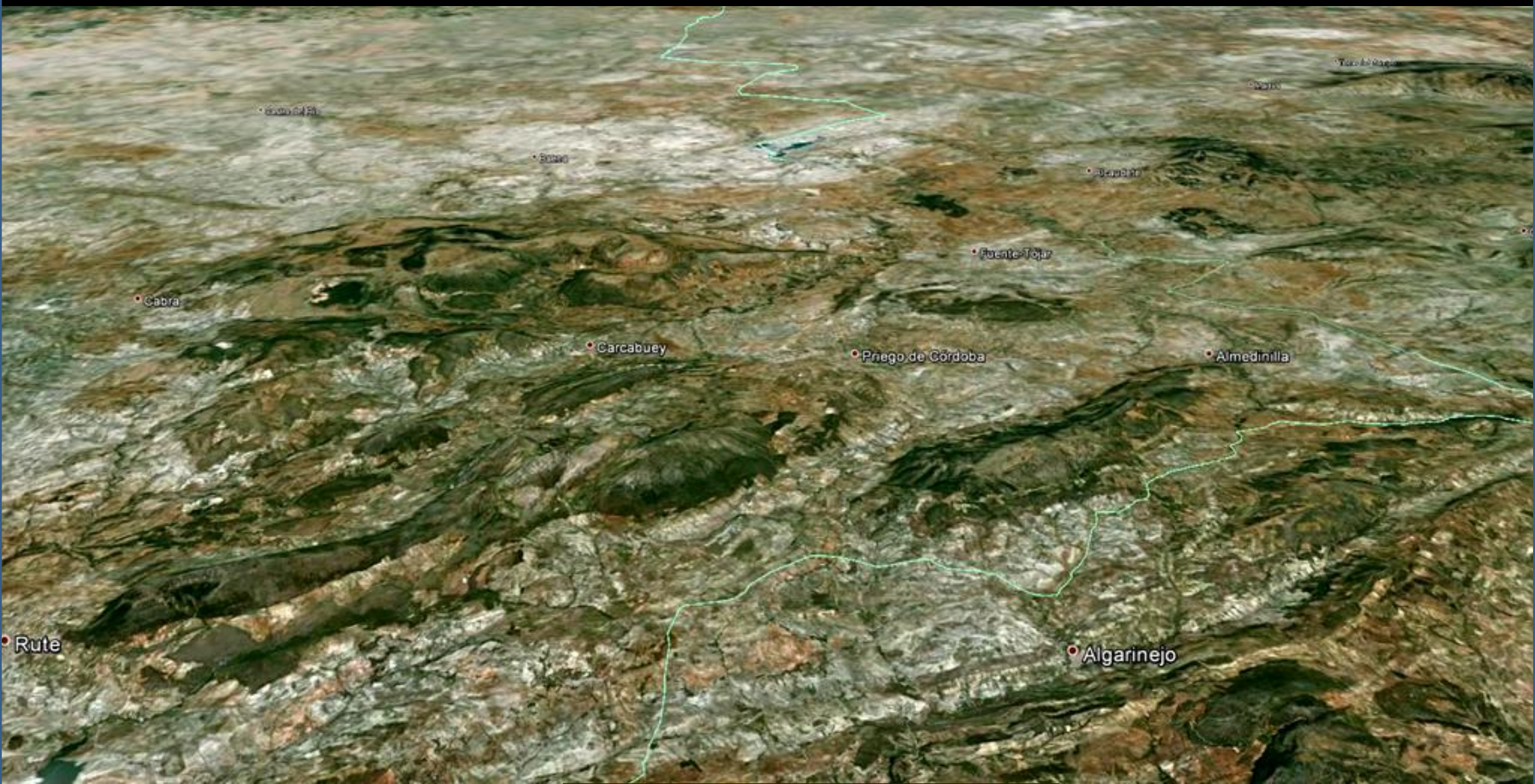
Perspectiva desde el S.-relieve realizado- SE de Córdoba.
